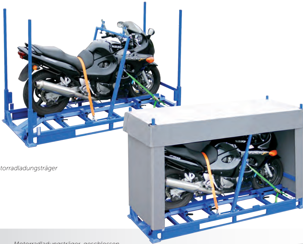
Motorradladungsträger, geschlossen
